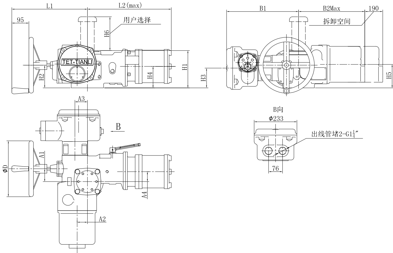
SMC-00~2整体型外形尺寸
